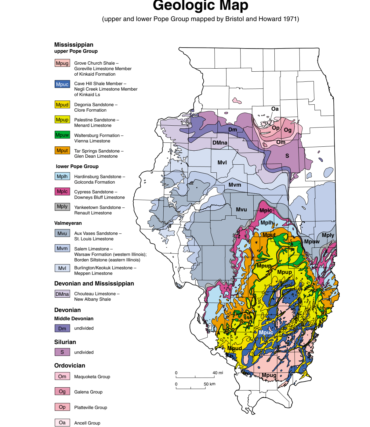
Sub-Absaroka (Sub-Pennsylvanian) Geologic Map
