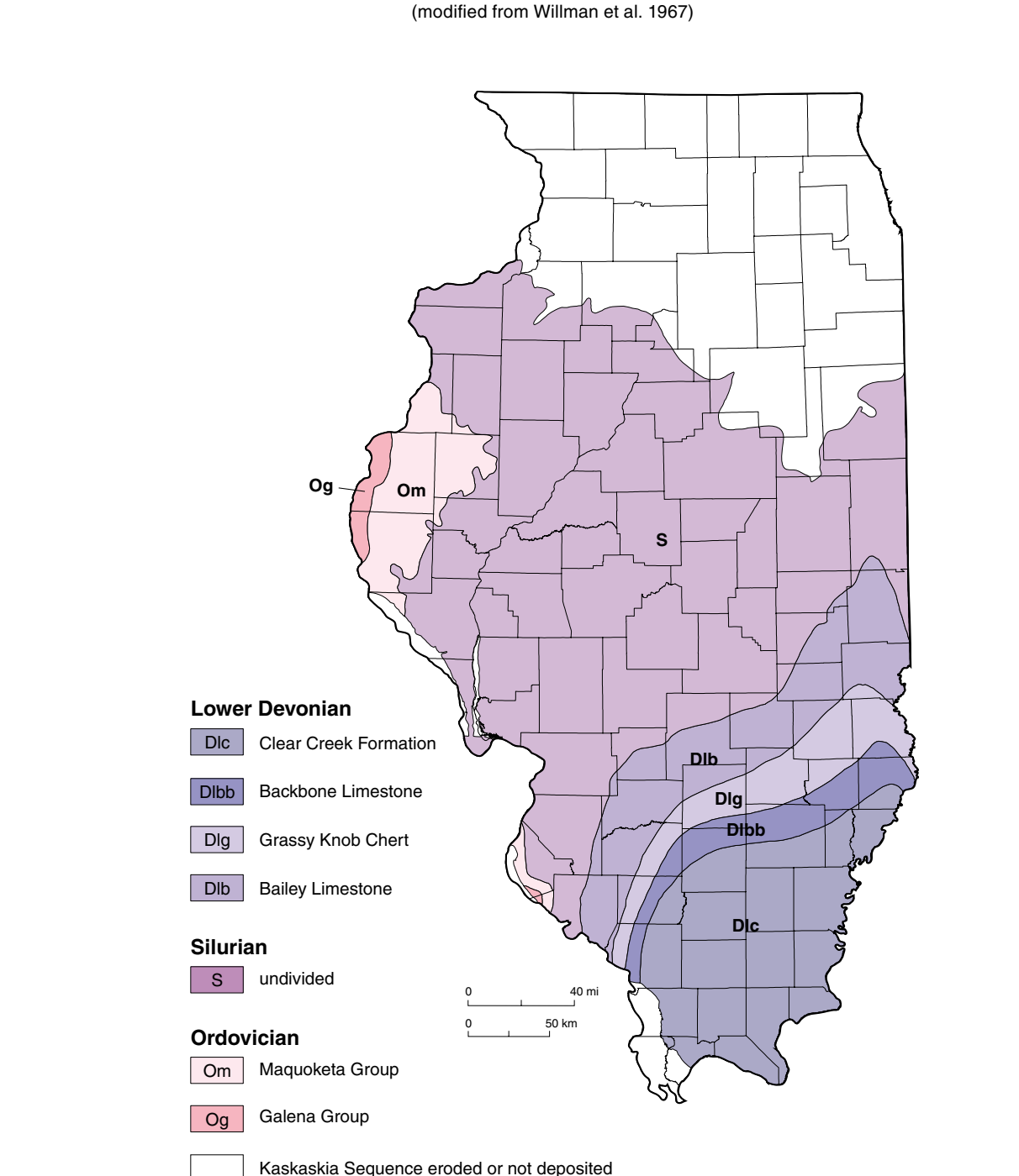
Sub-Kaskaskia Geologic Map
